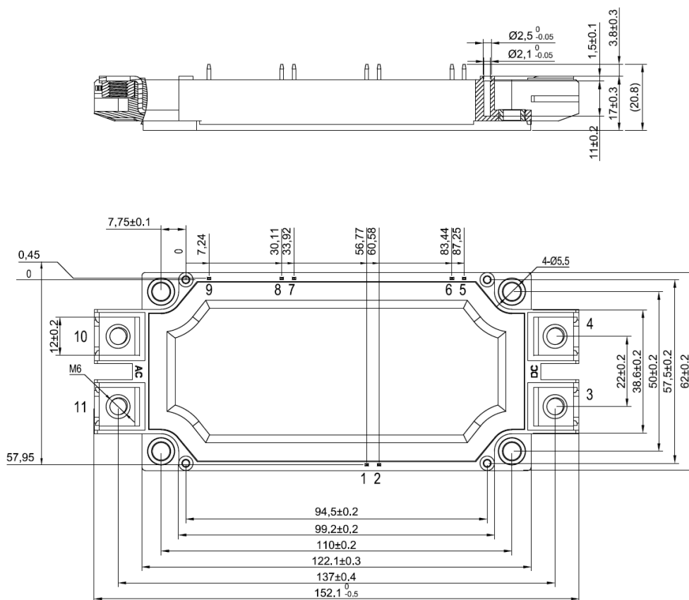
外形尺寸 Outline Drawing
