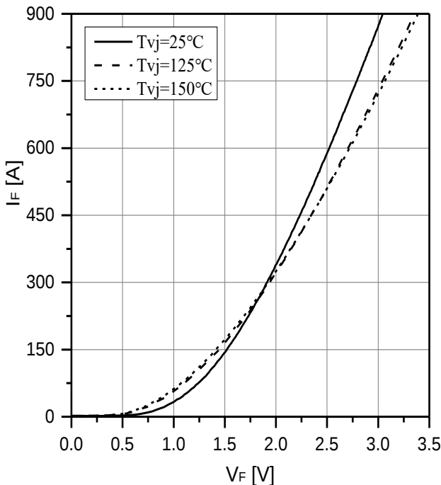
图8 二极管正向特性 Fig.8 Diode Forward Characteristic I_F vs V_F
